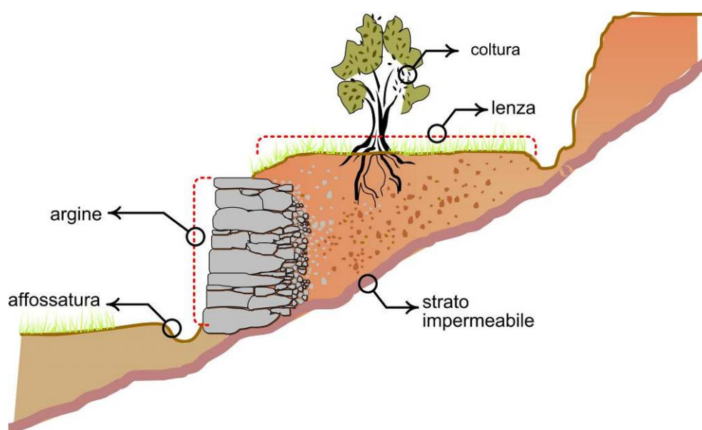
Schema degli elementi costitutivi del terrazzamento.
