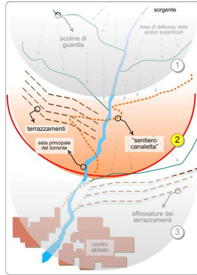
Muri di sostegno della viabilità e percorsi idraulici
