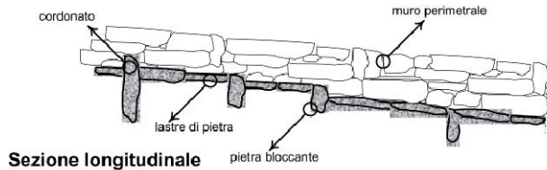
Sezione longitudinale
