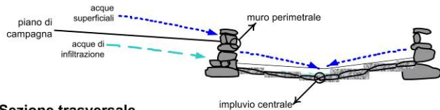
Sezione trasversale
