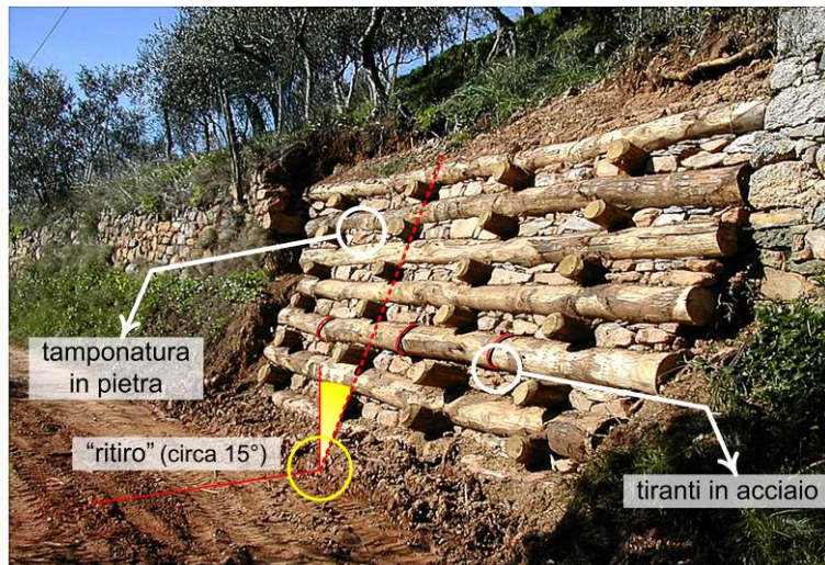
Struttura tipo di un intervento misto
