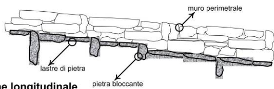
Sezione longitudinale
