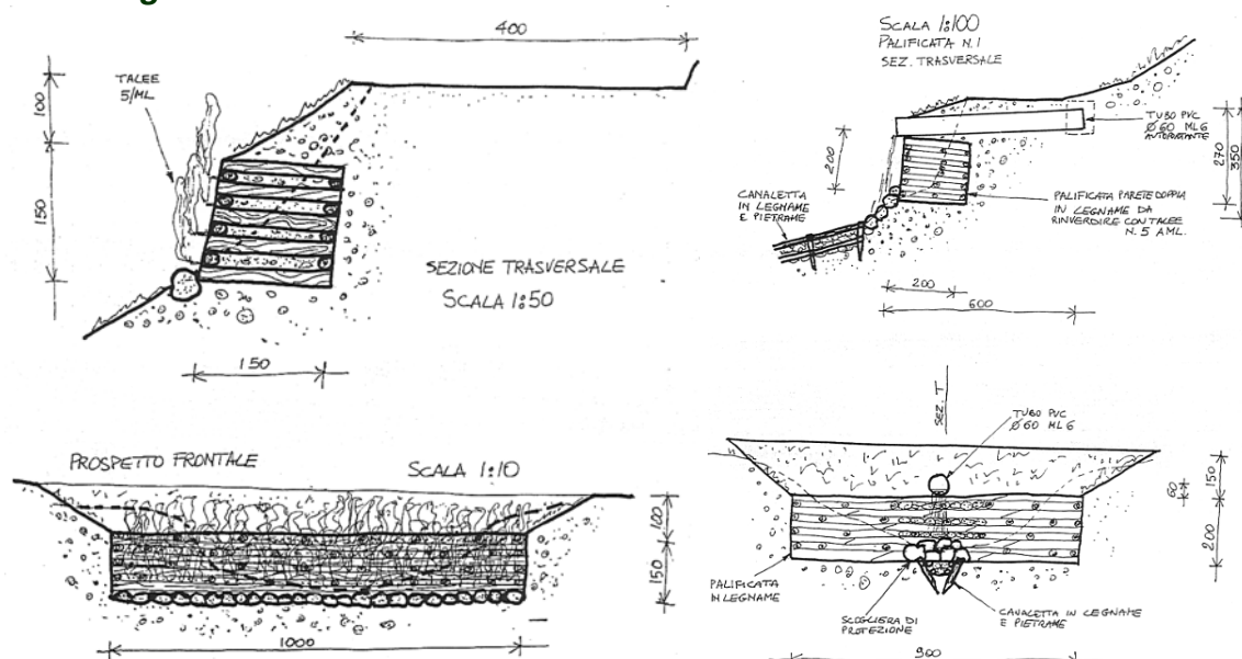
Sezioni tipo dei principali interventi [Schemi: Cooperativa Agriturstica Lungomonte].
