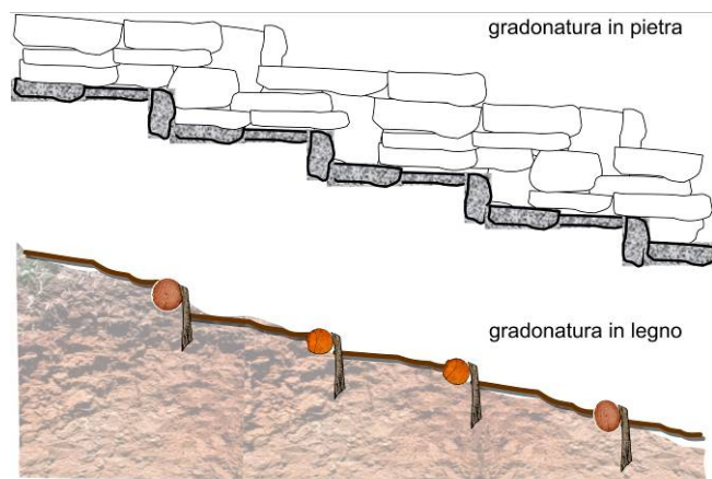
Sezione longitudinale
