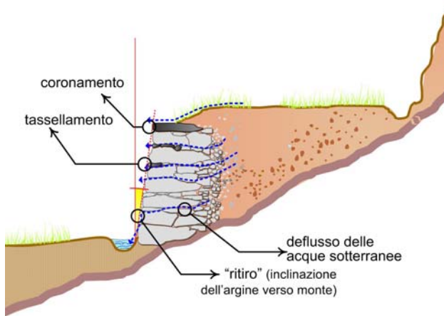
Schema visto in sezione e in foto frontale
