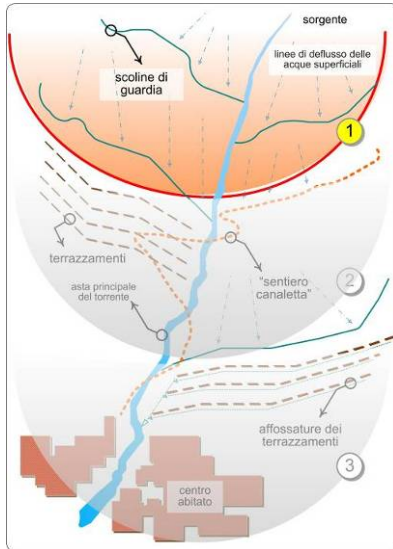
Scoline di guardia e canali collettori
